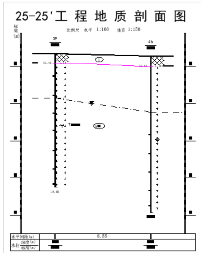
图 2-2 工程地质剖面图
