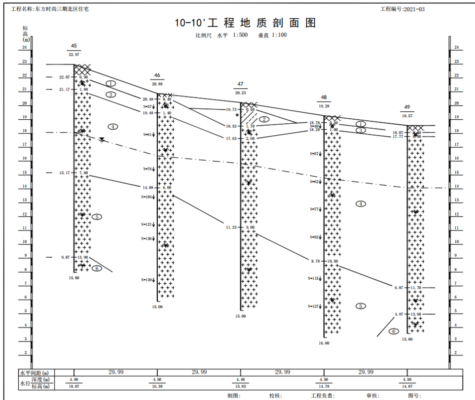
图 2-2 地块地质剖面图 1
